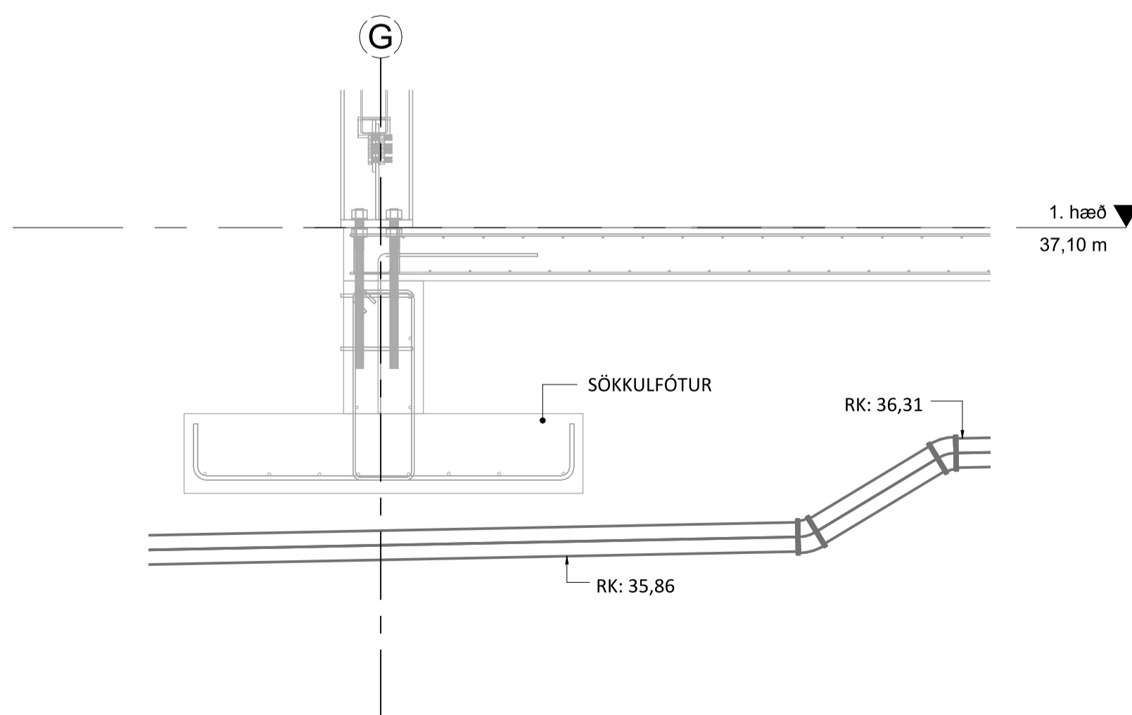
1-2 SNID VIÐ LAGER 1 : 20
