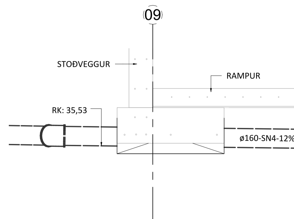
1-3 LÖGN UNDIR STÖÐVEGG 1 : 20
